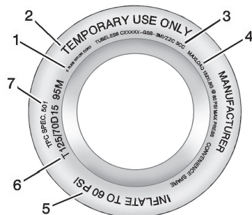
컴팩트 스페어 타이어의 예
