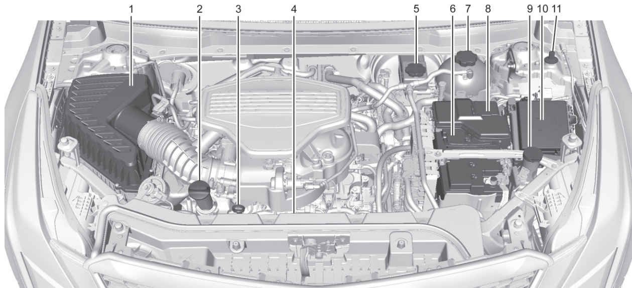
3.6L V6 엔진
