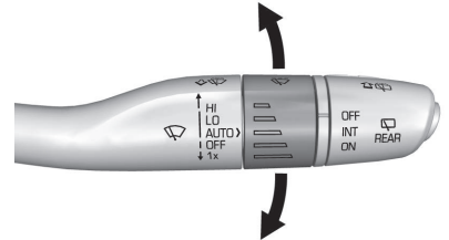
레인센서가 있는 앞유리 와이퍼(AUTO 모드)
