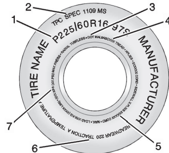
승용차(P-Metric)의 타이어 측벽에 나오는 정보의 예
