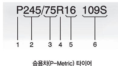
승용차(P-Metric) 타이어
