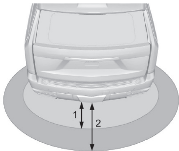
1. 인증 구역(1m) 2. 접근 구역(3m)
