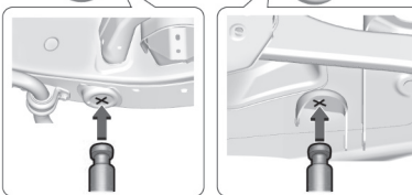
잭 받침부
