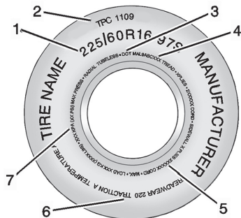
승용차의 타이어 측벽에 나오는 정보의 예
